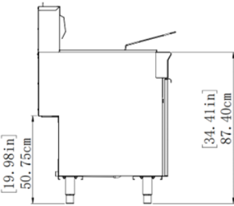
MODEL : TFDF-50-2V
